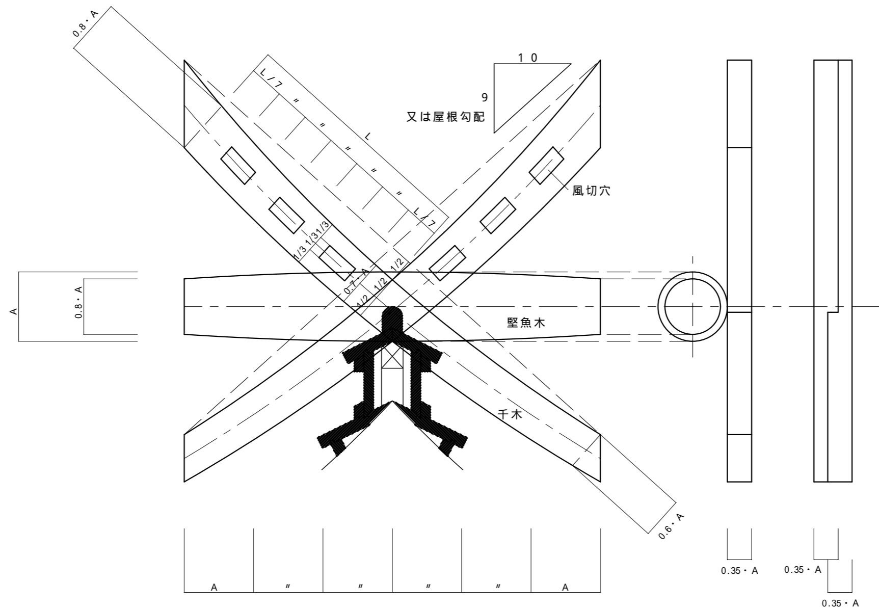
一間社流造 堅魚木・千木詳細図(2) 1/10
