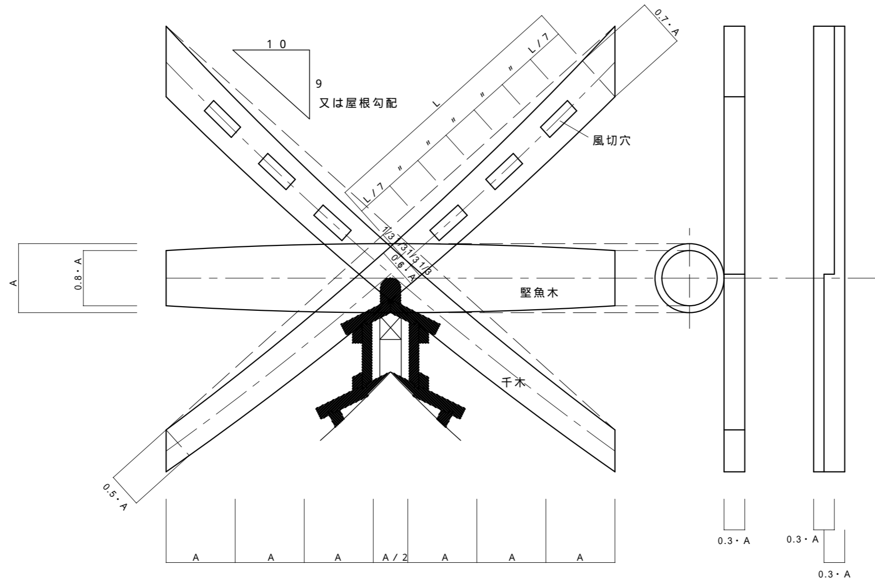
一間社流造 堅魚木・千木詳細図(1) 1/10
