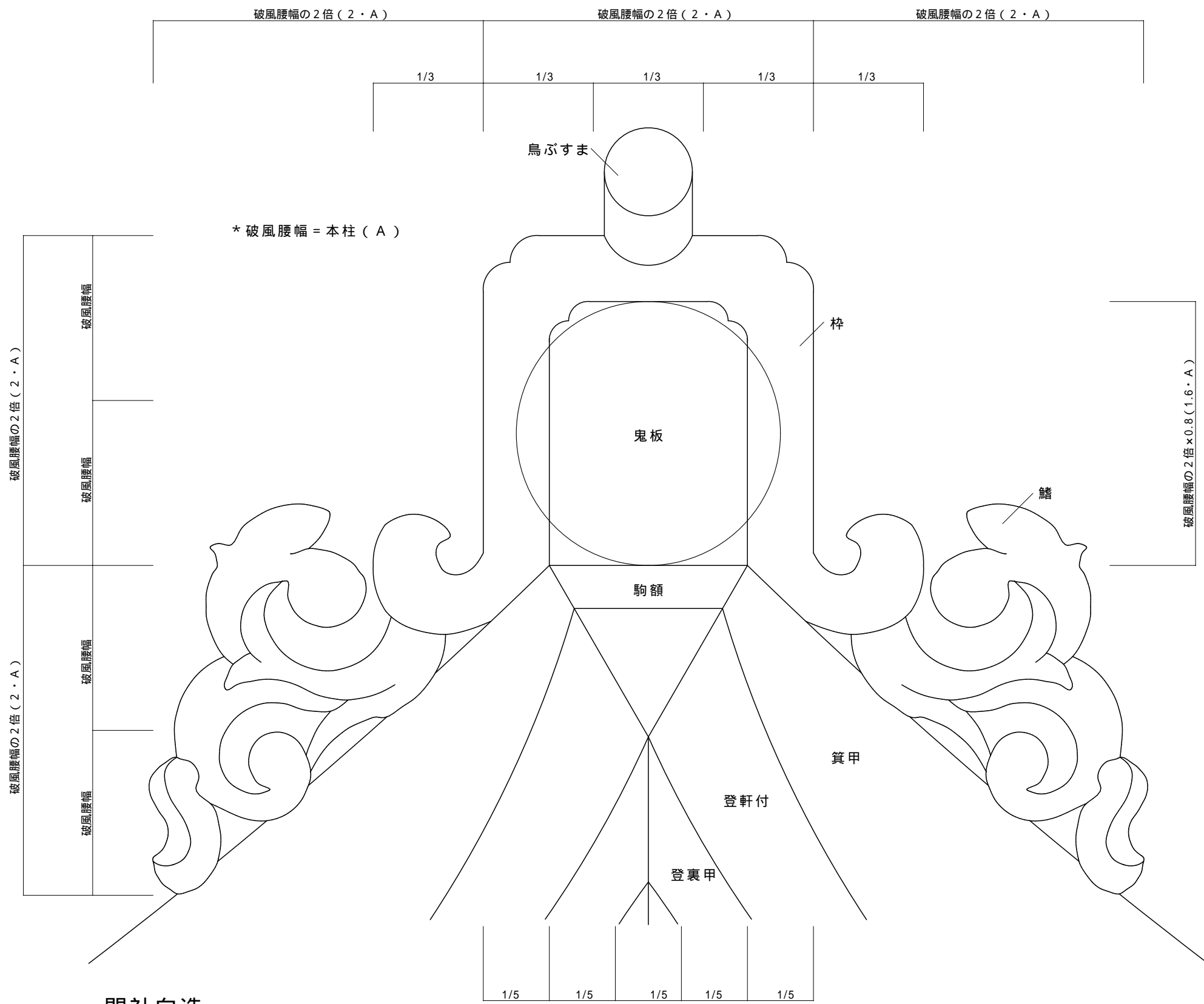
鬼板、鰭詳細図 1 / 5
